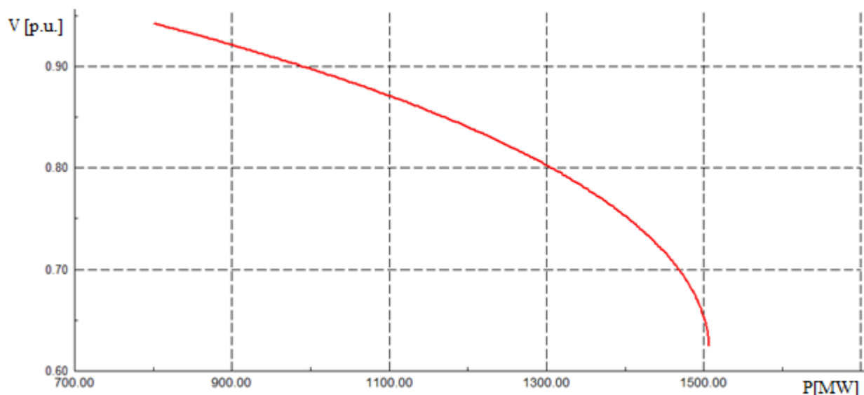
Slika 4.4. P-V krivulja faktora snage \cos\varphi = 0.9 (ind)
