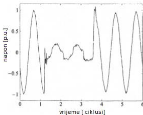
Slika 4.4. Naponski propad uzrokovan kratkim spojem [9]
