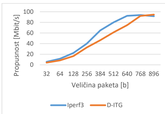
Slika 5.13. TCP propusnost
