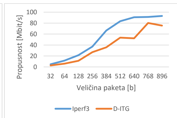
Slika 5.14. UDP propusnost
