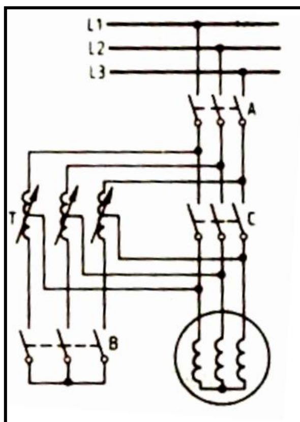
Slika 2.9. Pokretanje elektromotora autotransformatorom [5]
