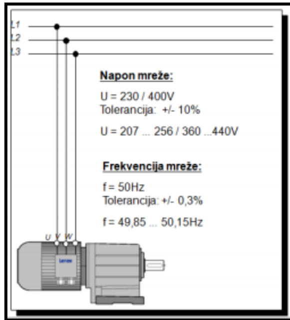
Slika 3.7. Motor spojen bez pretvarača [10]
