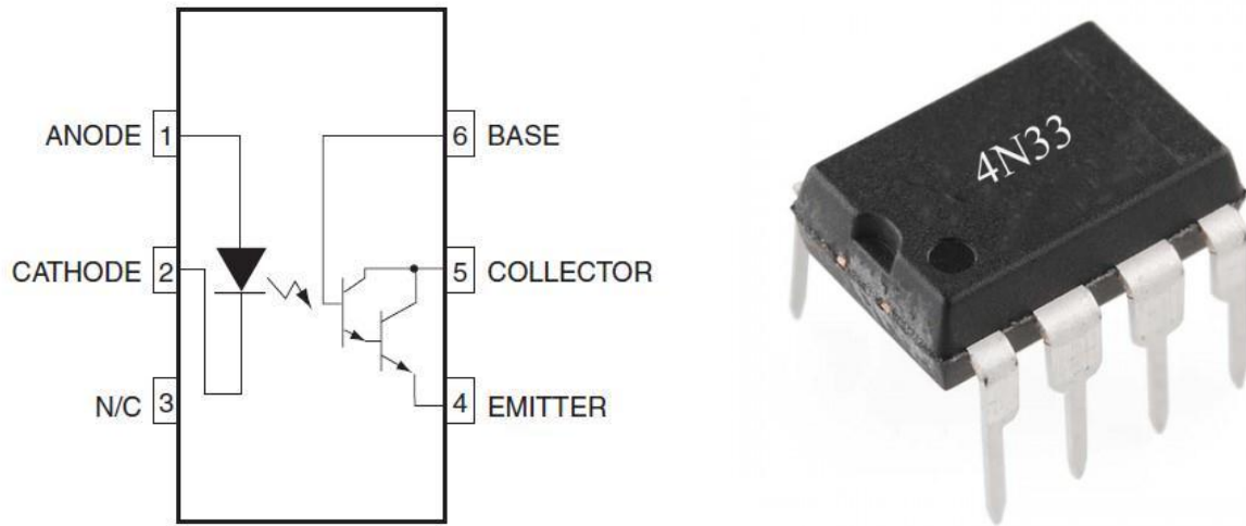
Sl. 4.10. Unutarnja shema i realni izgled optoizolatora 4N33 [5].
