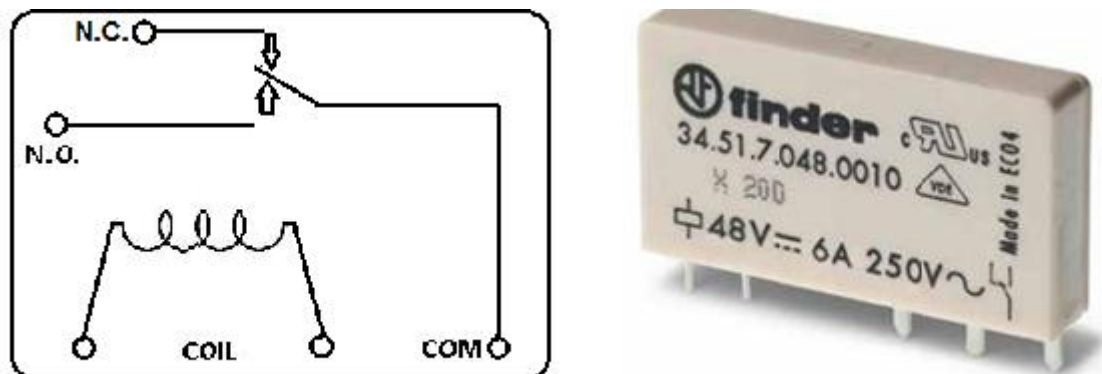
Sl. 4.11. Shema jednopolnog releja i realna izvedba releja [6].
