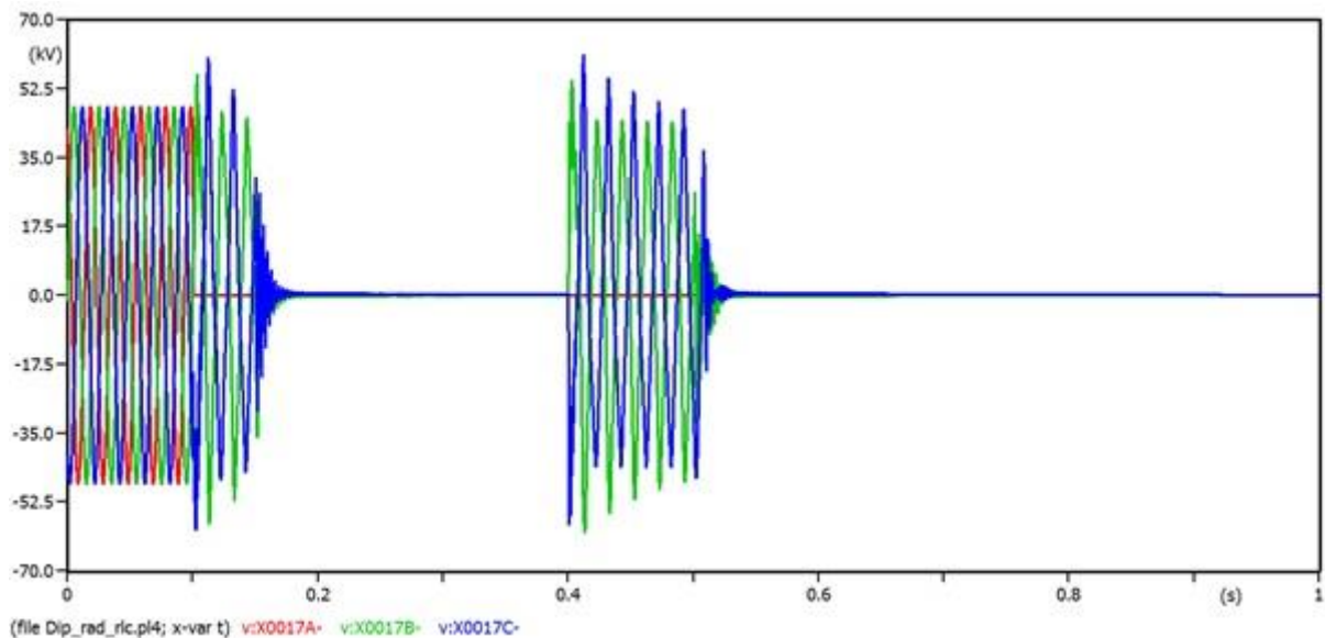
Sl. 5.10. Valni oblici napona pojedinih faza na mjestu kvara pri jednofaznom kratkom spoju
