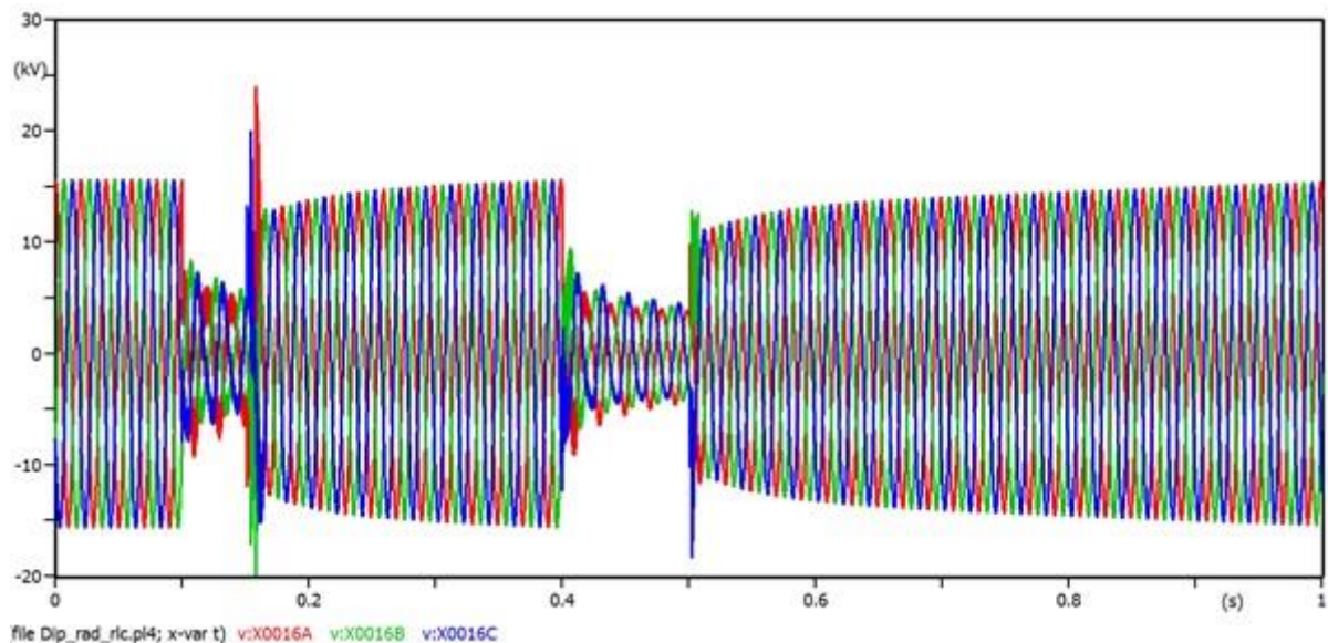
Sl. 5.12. Valni oblici napona pojedinih faza generatora pri trofaznom kratkom spoju
