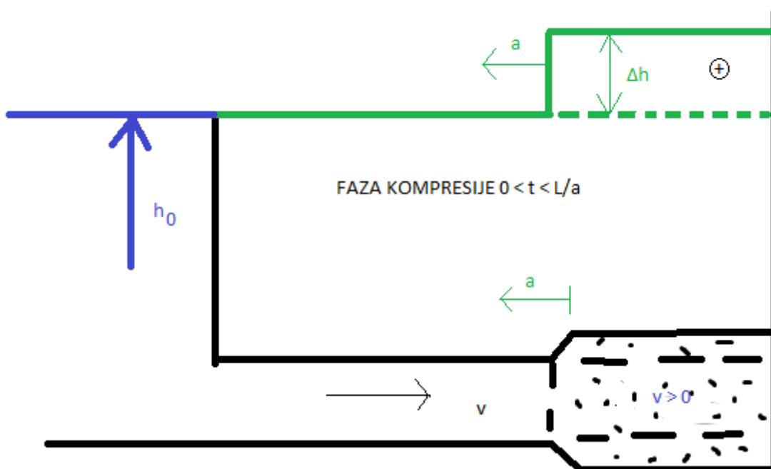
Sl. 5.1.b) Faze propagacije vodnog udara
