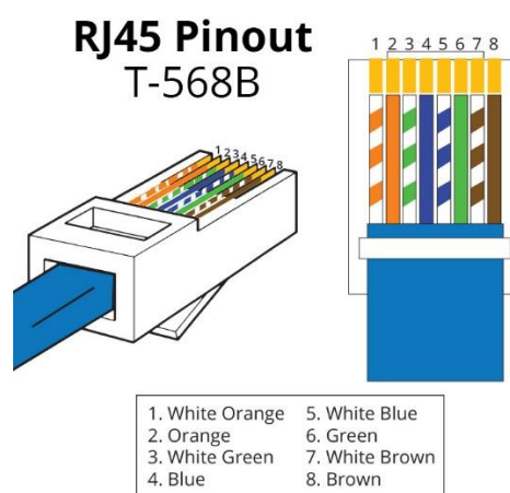
Slika 4.2.2. T-568B standard [13]
