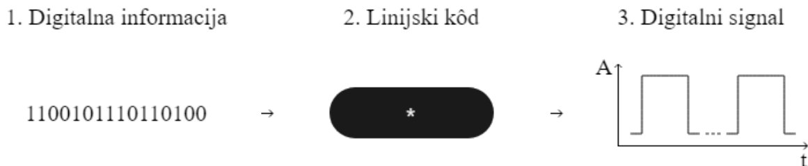
Slika 2.1. Uloga linijskog koda u komunikacijskom kanalu
