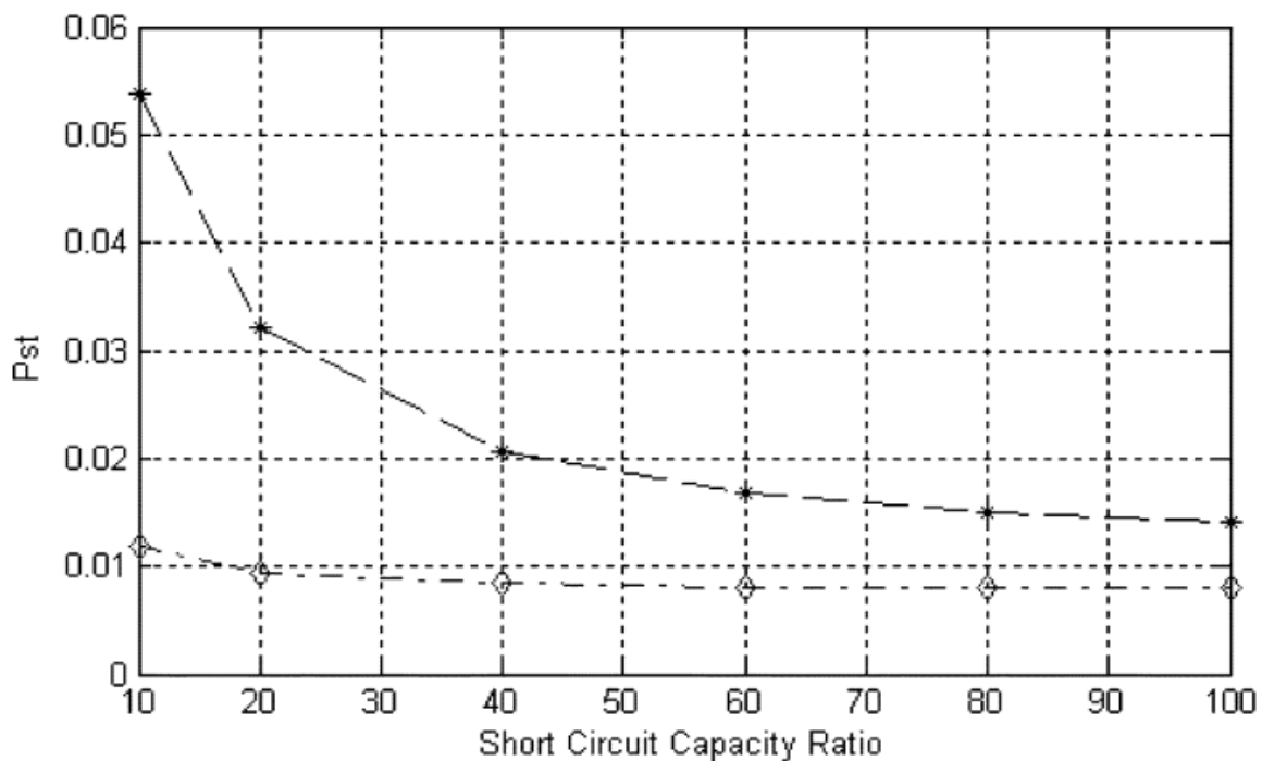
Slika 5.13. Kratkotrajna jačina treperenja u ovisnosti o kapacitetu kratkog spoja u turbulencije ( v=18 m/s, In = 0,1 , SCR = 20 , \psi k= 63: 4349^\circ , normalan rad (zvjezdica), s kontrolom jalove snage (dijamant), preuzeto iz [12]).
