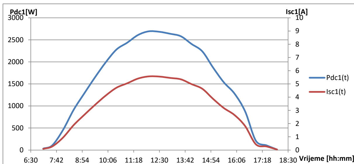
Slika 3.6. Odnos promjene istosmjerne snage i struje kratkog spoja jednog FN niza u periodu jednog dana
