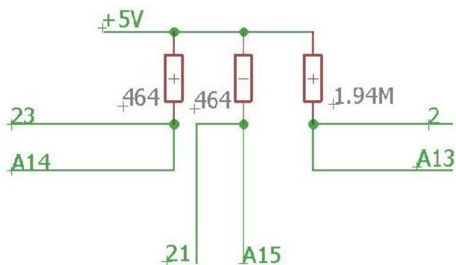
SI 3.7. Shema spajanja naponskog djelila
