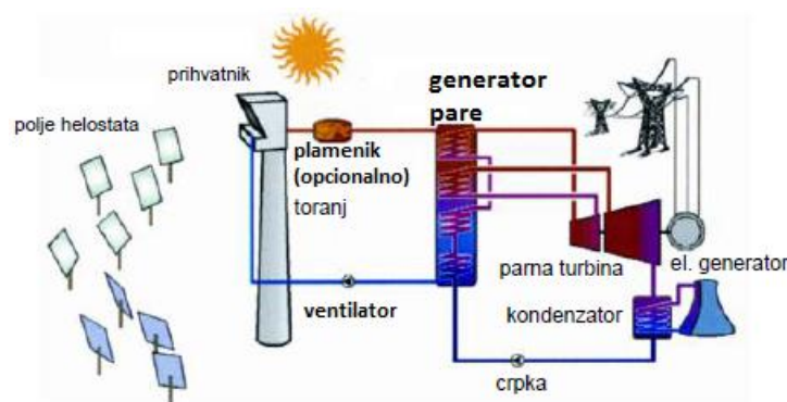
SI.3.3. Shema hibridne solarne termoelektrane s otvorenim volumetrijskim prijamnikom [11].
