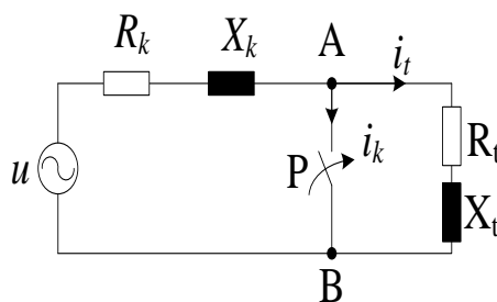
Sl.3.1. Pojednostavljena shema strujnog kruga
