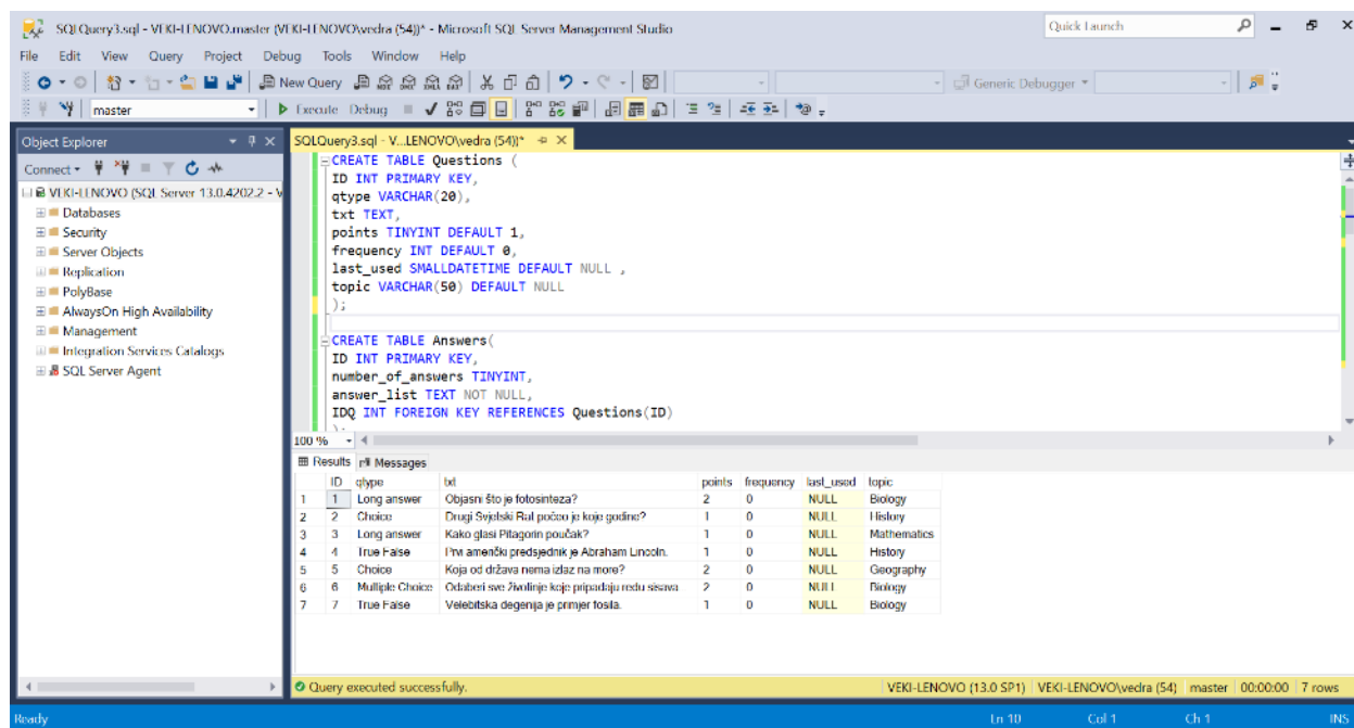
Sl. 2.2. Izgled sučelja programa Microsoft SQL Server Management Studio
