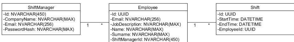
Sl. 3.19 UML dijagram tablica
