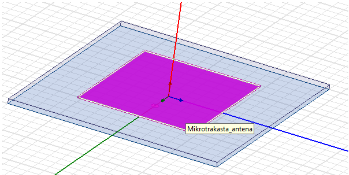
SI. 5.2.15. Prikaz Mikrotrakaste antene koja se nalazi na supstratu
