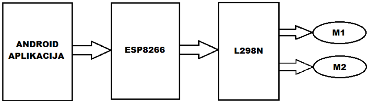
Slika 10. Funkcijski dijagram sustava
