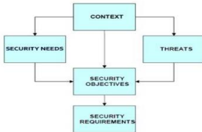
Slika 3.9. Metodologija EBIOS-a [8]
