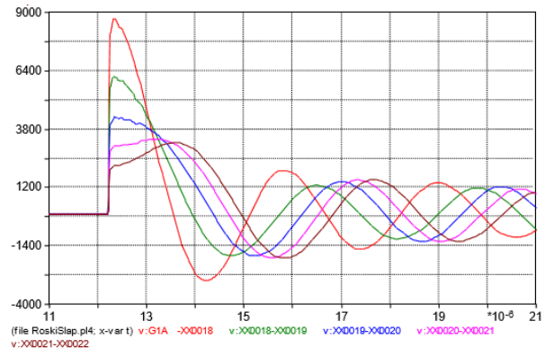
Sl. 6.20. Valni oblik napona na prvim pet zavoja prvog svitka ( V1_{max}=8,73 kV; V2_{max}=6,17 kV; V3_{max}=4,36 kV; V4_{max}=3,36 kV; V5_{max}=3,21 kV)
