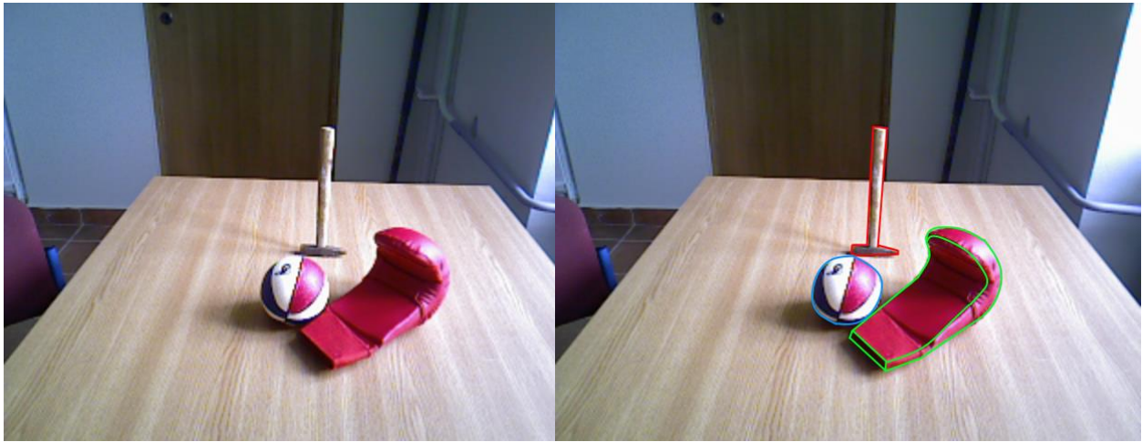
Slika 8.11.a Ulazna slika
