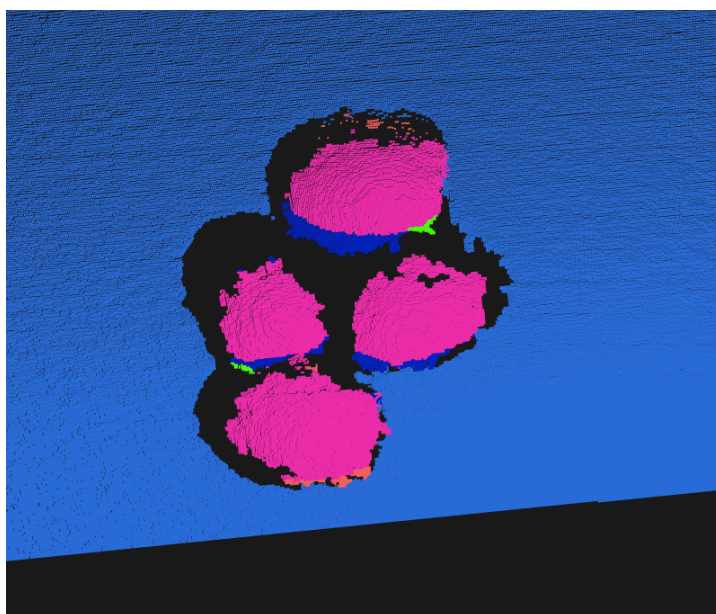
Slika 8.20.c Segmentirana slika
