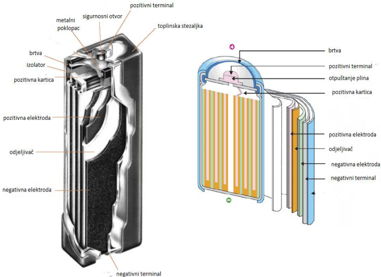
Slika 3.6. Shema prizmatske (lijevo) i spiralne (desno) Ni-MH baterije [3]
