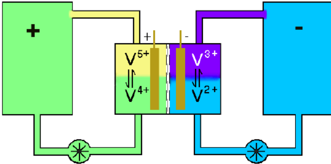
Slika 3.10. Shema vanadij redoks baterije [3]
