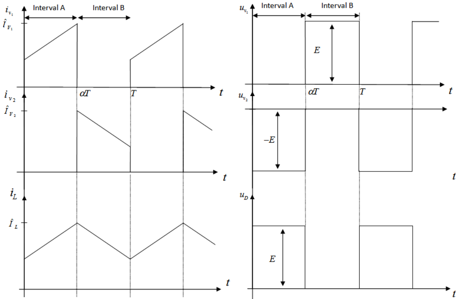
Slika 3.4.: Valni oblici struja i napona
