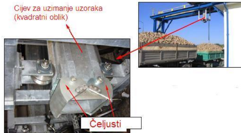
Slika 5.5 Čeljusti sonde za uzimanje uzoraka [2]
