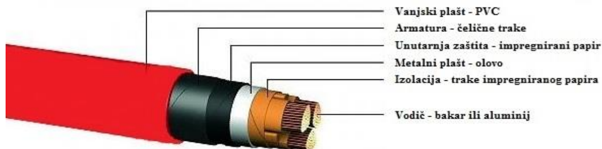
Sl. 4.3. Energetski kabal IPO 14, IPO 14-A [5]
