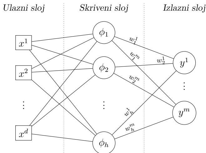
Slika 5.1: Uobičajena struktura RBFN klasifikatora
