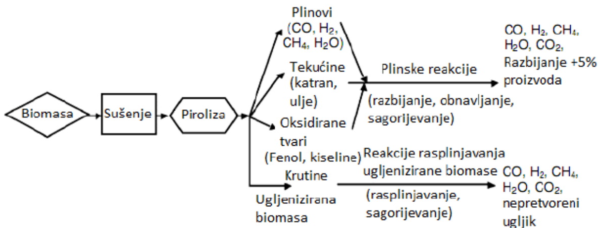
Slika 3.2. Smjerovi rasplinjavanja [6]
