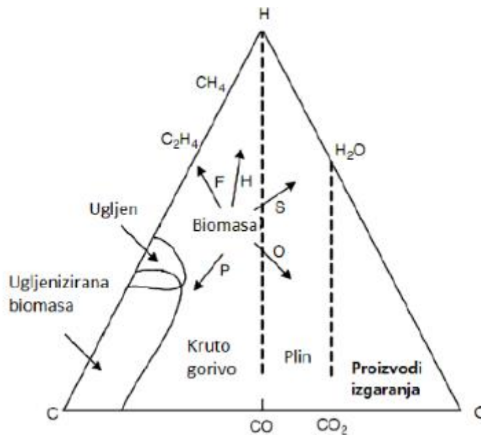
Slika 3.1. Proces rasplinjavanja, trostruki dijagram (C-H-O) [6]
