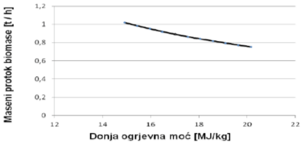
Slika 3.7. Ovisnost masenog protoka potrebne biomase o donjoj ogrjevnoj moći [7]
