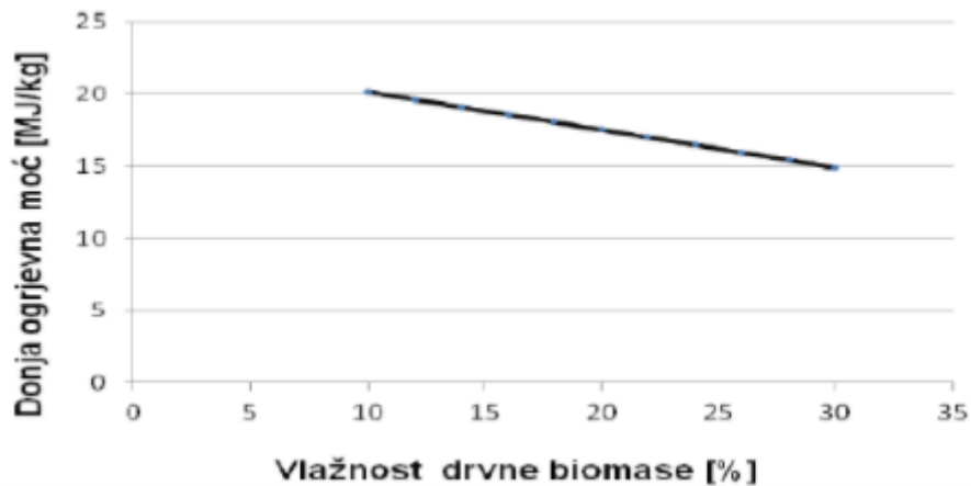
Slika 3.8. Ovisnost donje ogrjevne moći drvene biomase o vlažnosti [7]
