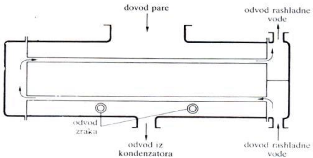
Slika 4.6. Skica kondenzatora [12]
