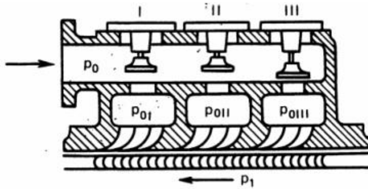
Slika 6.3 Regулacija s više ventila[15]
