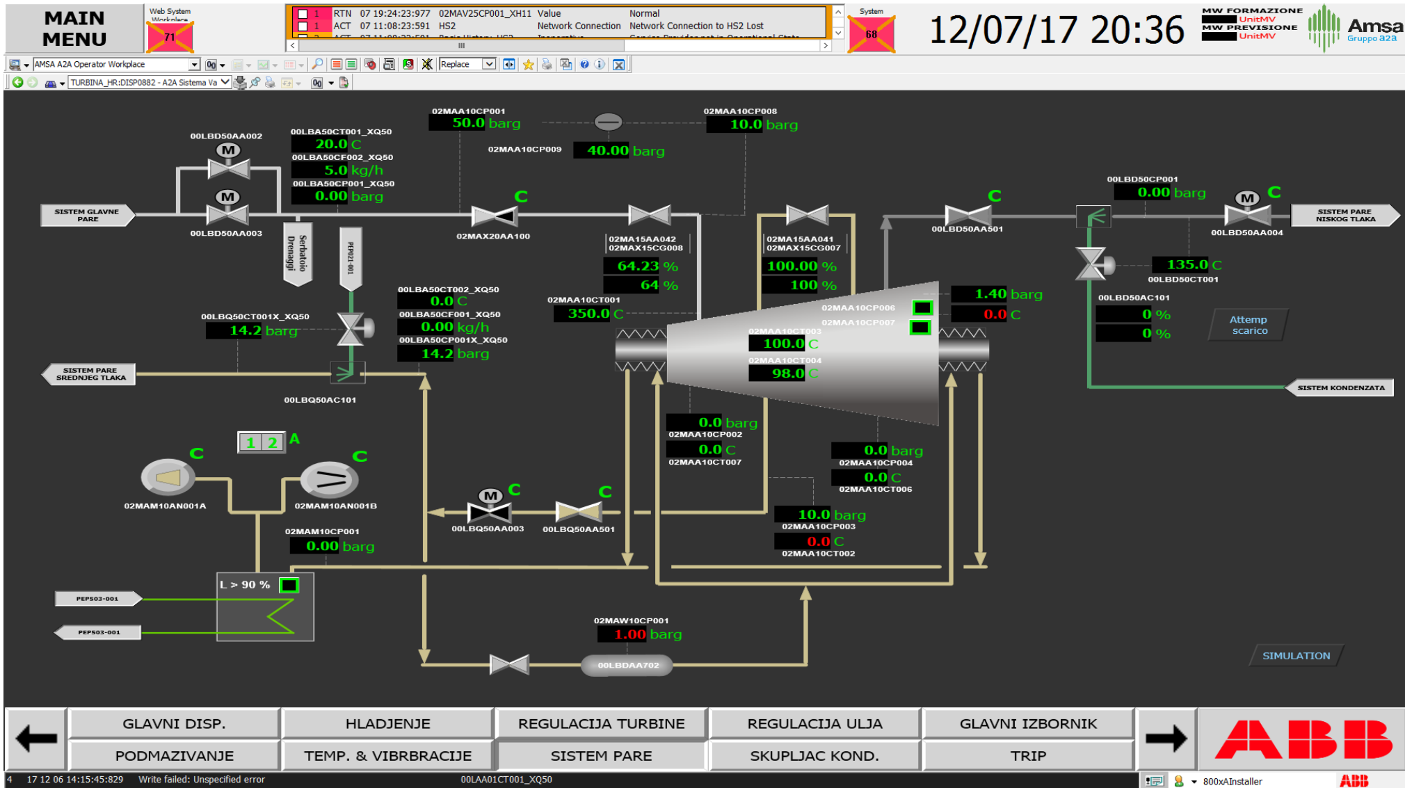
Slika 7.8 Sistem toka pare
