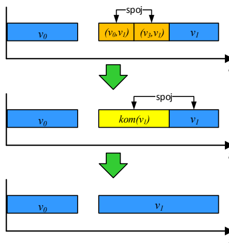
Slika 4.16: Postupak SKO.
