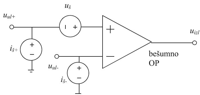
Slika 3.11. Izvori šuma u operacijskom pojačalu
