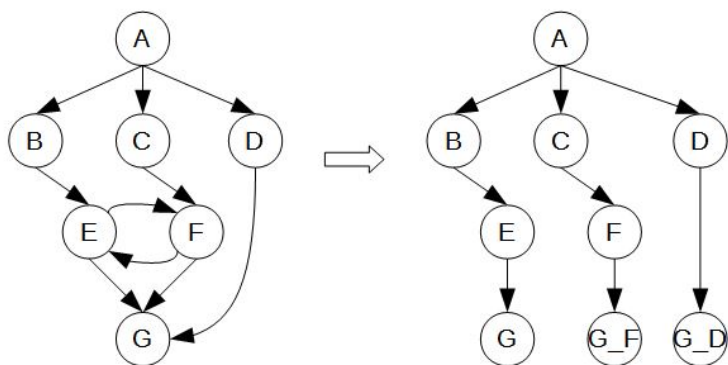
Slika 6.11: Podpravilo 4
