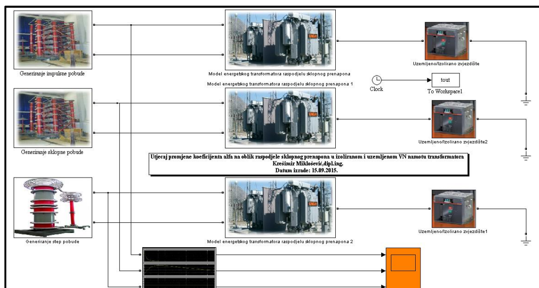
Slika 6.16. Simulacijski model za analizu utjecaja promjene koeficijenta \alpha na oblik raspodjele sklopnog prenapona u uzemljenom i izoliranom namotu
