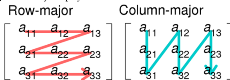
Sl. 2.2. Row-major redosljed i Column-major redosljed metode spremanja višedimenzionalnih polja, prema [8].
