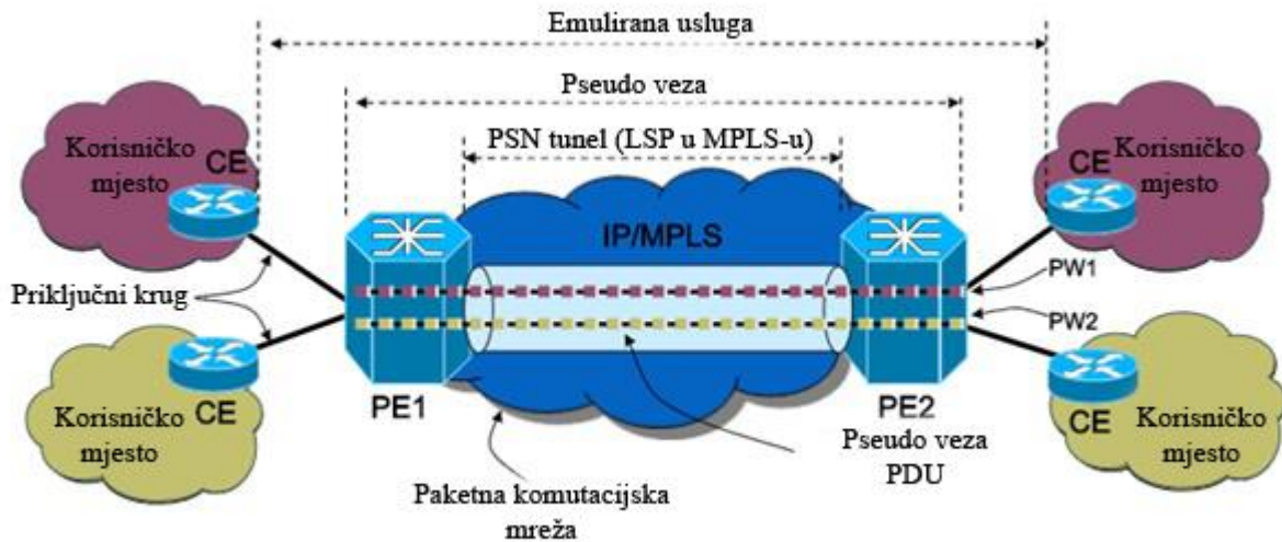
Slika 5.8. PWE3 model [50]
