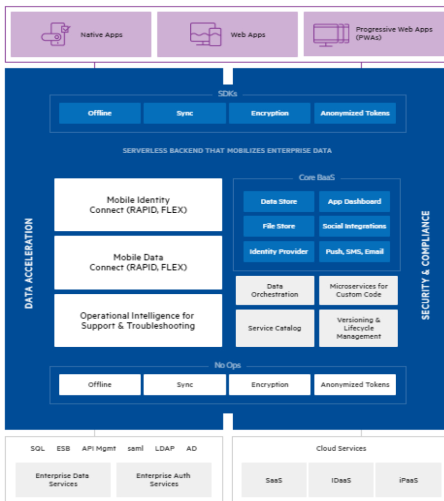
SI. 3.3. Blokovski dijagram arhitekture sustava Kinvey [22]
