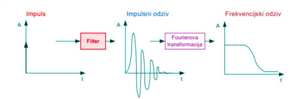
Sl. 2.1. Impulsni i frekvencijski odziv filtera[3]
