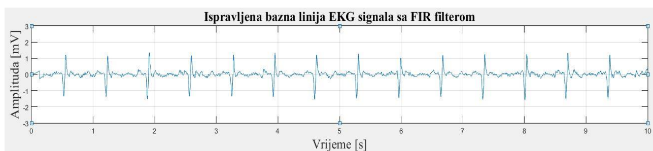
SI.4.9. Ispravljena bazna linija KEG signala sa FIR filterom
