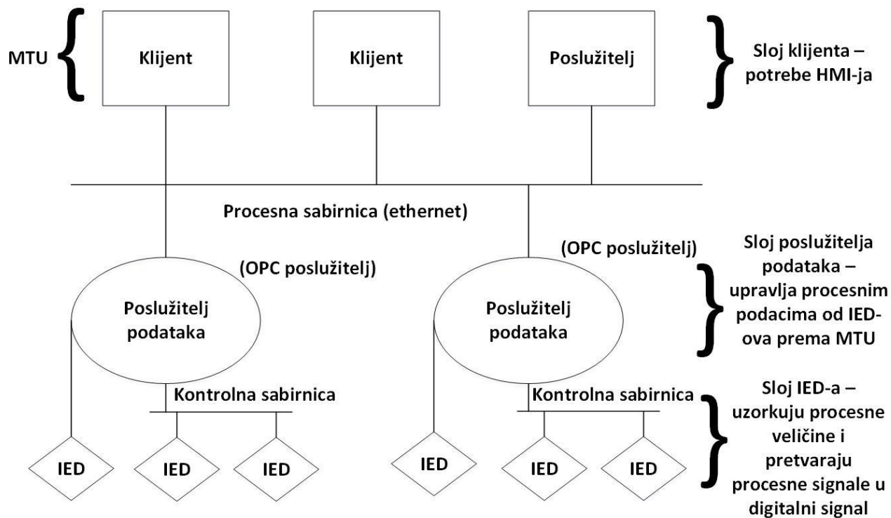
Slika 2.3. Sklopovska struktura SCADA-e.
