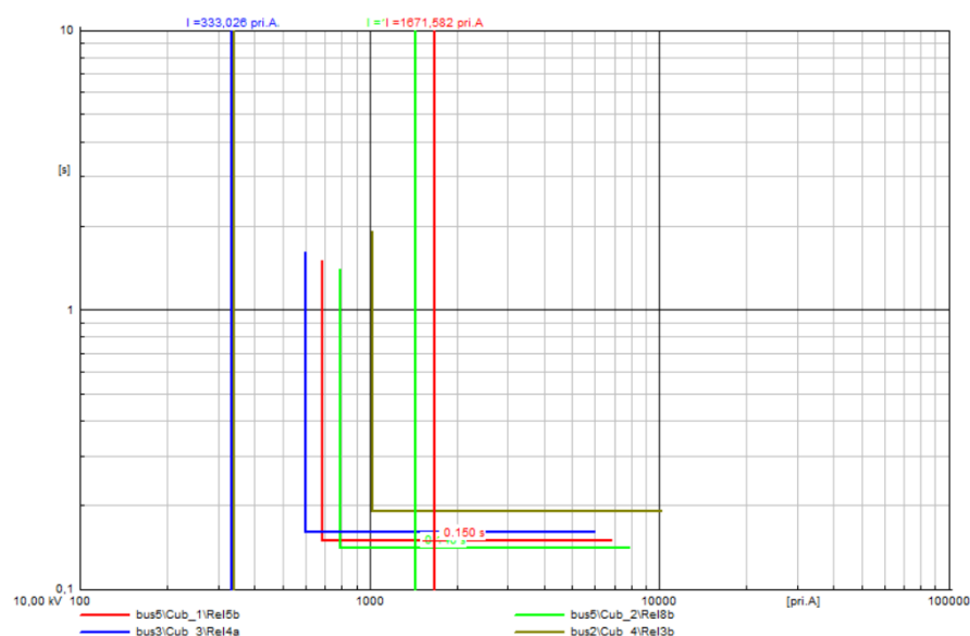
Sl. 6.66. I-t dijagrami releja za kratki spoj na sabirnici bus5 uz priključene tri VE (doprinos struji KS I_{1,1In} ) na sabirnicama bus4, bus5 i bus6
