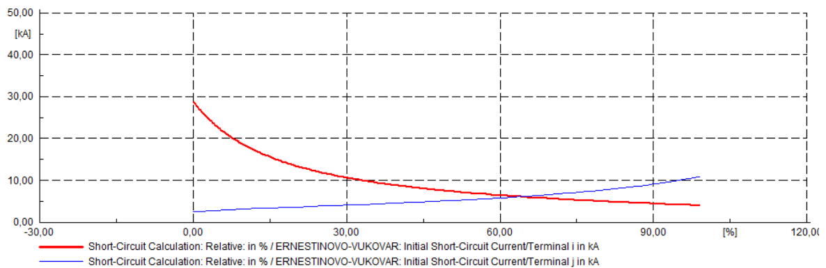
Slika 6.14. Rezultati skripte izvedene na vodu ERNESTINOVO-VUKOVAR (prvi VI)
