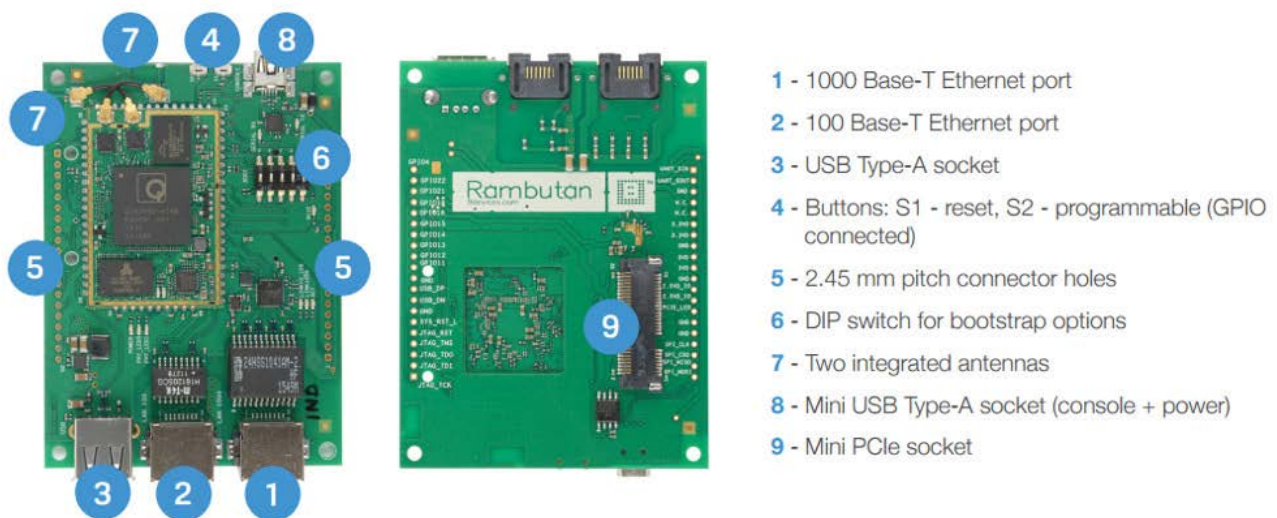
Slika 4.10. Rambutan uređaj [22]
