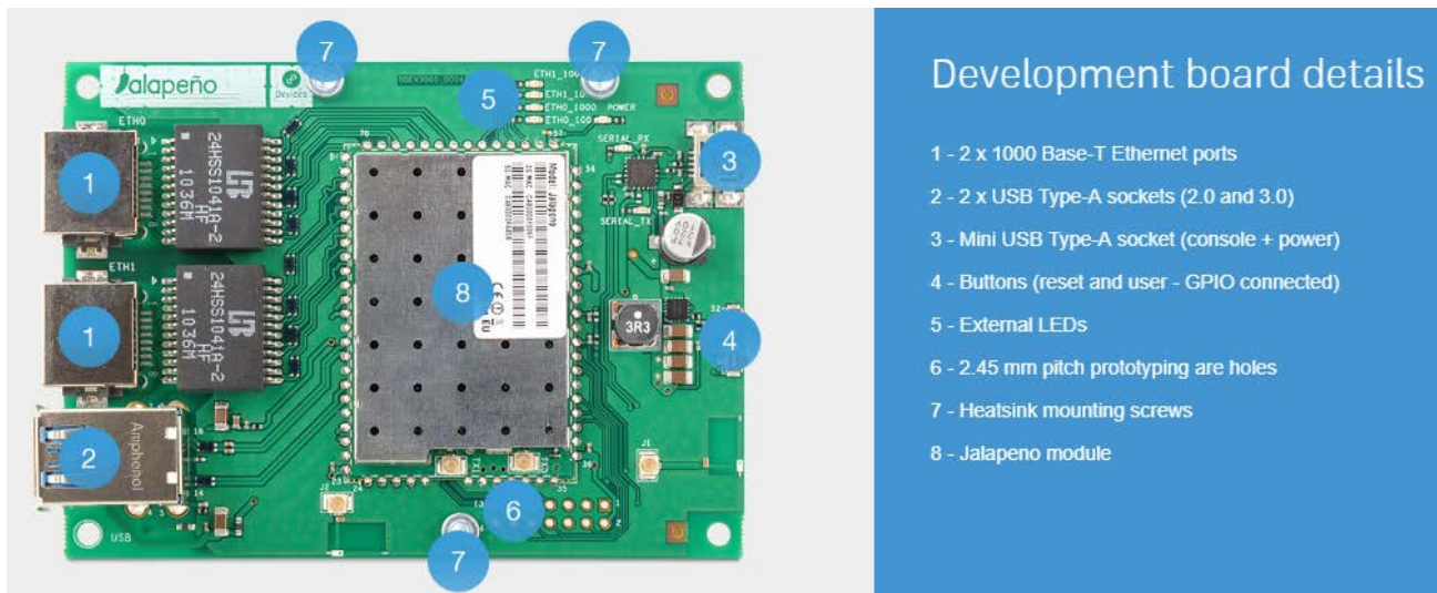
Slika 4.20. Jalapeno uređaj [23]
