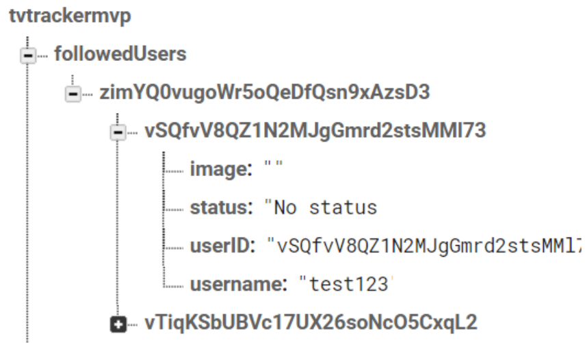
Slika 4.2. Prikaz grananja čvora followedUsers
