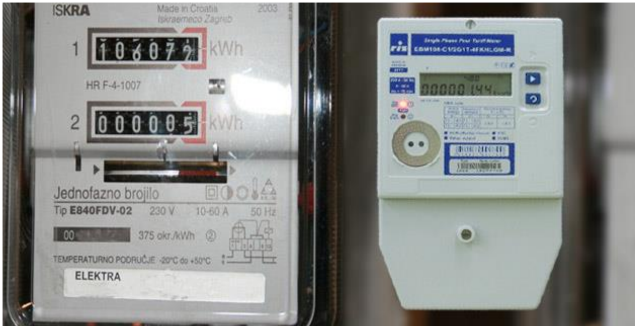
Slika 3.5. Prikaz elektromehaničkog i pametnog brojila [12]
