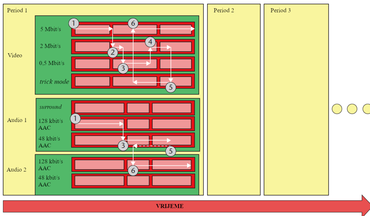
Slika 2.2. Slučaj korištenja dinamičkog prijenosa u MPEG-DASH-u [3]
