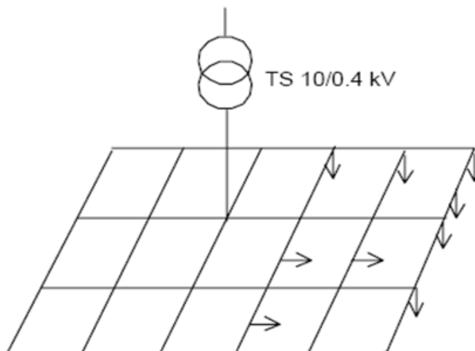
Slika 2.7. Uzamčena mreža sa jednim izvorom [4]
