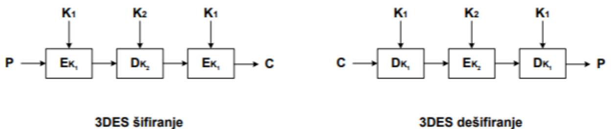
Slika 2.11. 3DES algoritam
