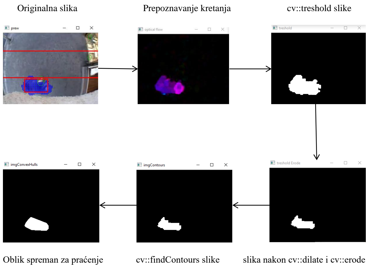
Sl.3.10. Faze obrade slike kod prepoznavanja i praćenja kretajućih oblika
